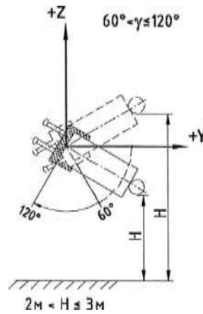
Рис. 3. Наклон пассажирских кресел наборов
